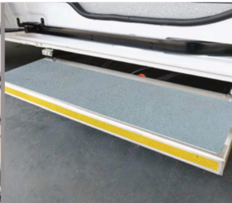
Peldaño de acero inoxidable y accionamiento eléctrico. Longitud 900 mm, capacidad de carga 150 Kg. Opción de asideros en la puerta corredera.
