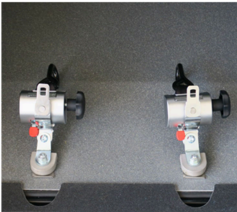
Retractor de acero inoxidable y cinturón para cada pasajero en silla de ruedas.
